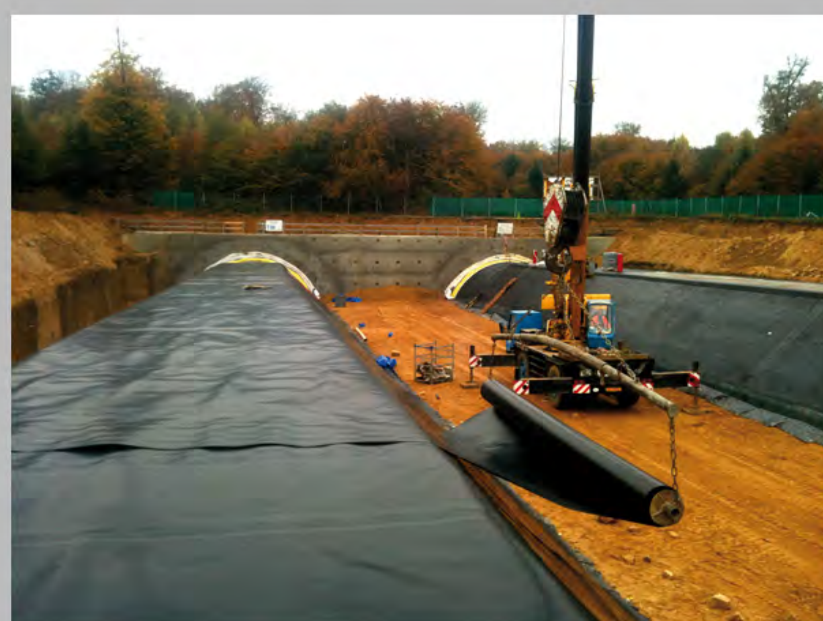
Tunnelabdichtung
