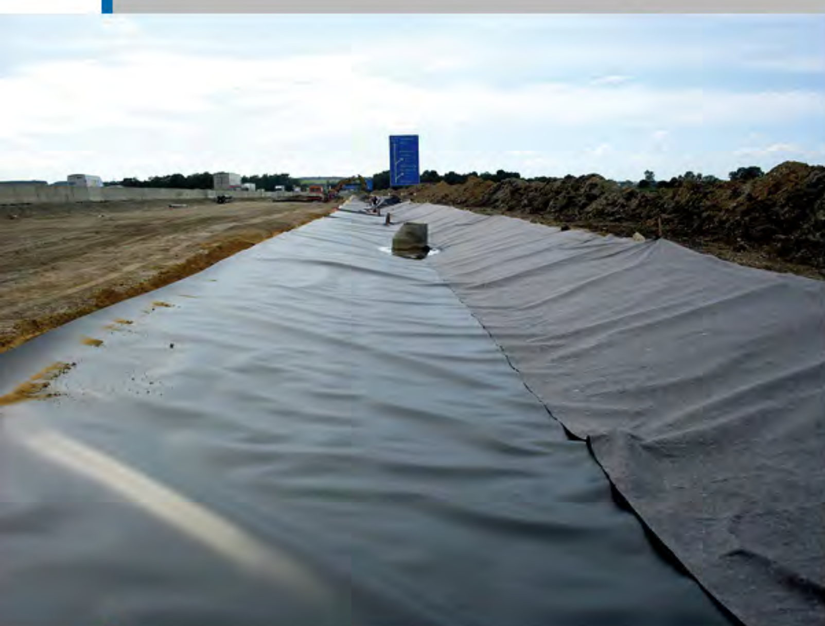
Autobahnabdichtung
